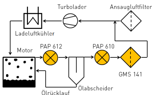
Beispiel: Integration des GMS 141 und der Photometer PAP 610 und PAP 612 in einem Motorenprüfstand
