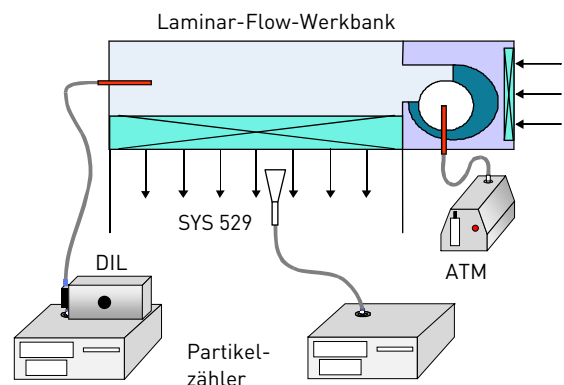
Abnahme einer Laminar-Flow-Werkbank mit den Topas-Geräten Aerosolgenerator ATM, Verdünnungssystem DIL, Probenahmesonde SYS 529 sowie dem Partikelzähler LAP 340
